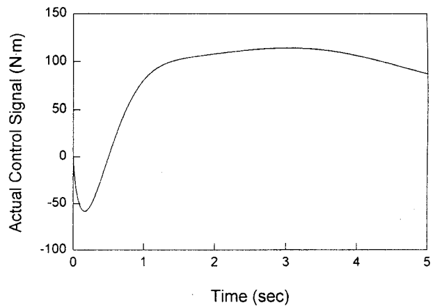
Figure 6. Actual control torque (τ)
