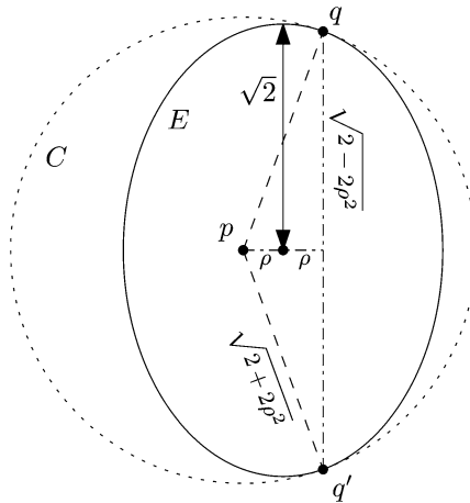
Fig. 3. Illustration for Lemma 7.
