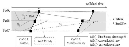
그림 3. Mattern의 알고리즘의 제약사항
