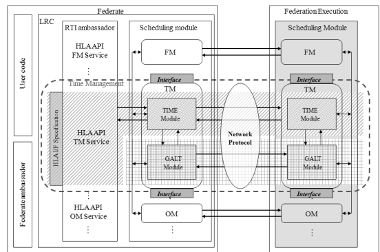
그림 5. 시간 관리 서비스 모듈의 프레임워크
