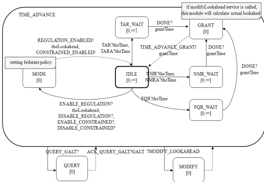
그림 6. LRC의 TIME 모듈의 상태천이도
