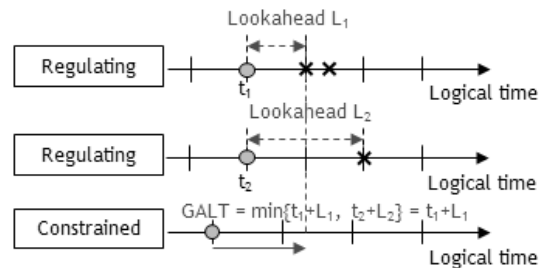
그림 1. 페더레이트 정책
