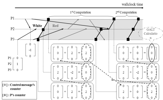
그림 2. Mattern의 알고리즘
