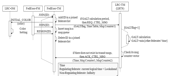
그림 7. GALT 계산의 시퀀스 다이어그램
