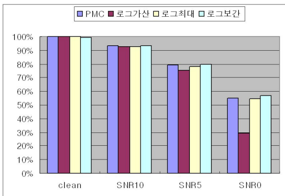
그림 3 단어 인식률 (%)
